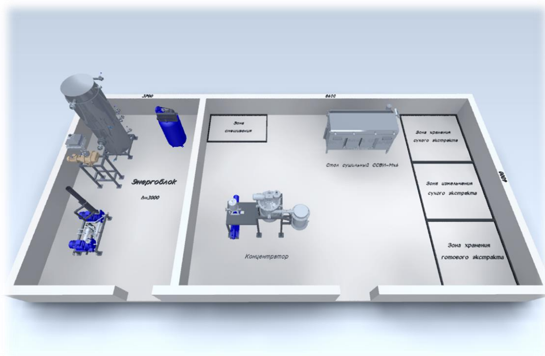
Вариант 3 – Один сушильный стол с концентратором и энергоблоком
