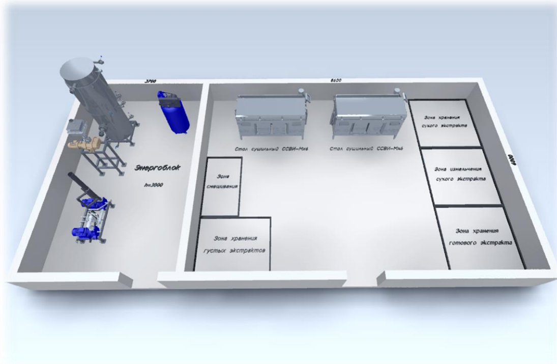
Вариант 2 – Два сушильных стола с энергоблоком
